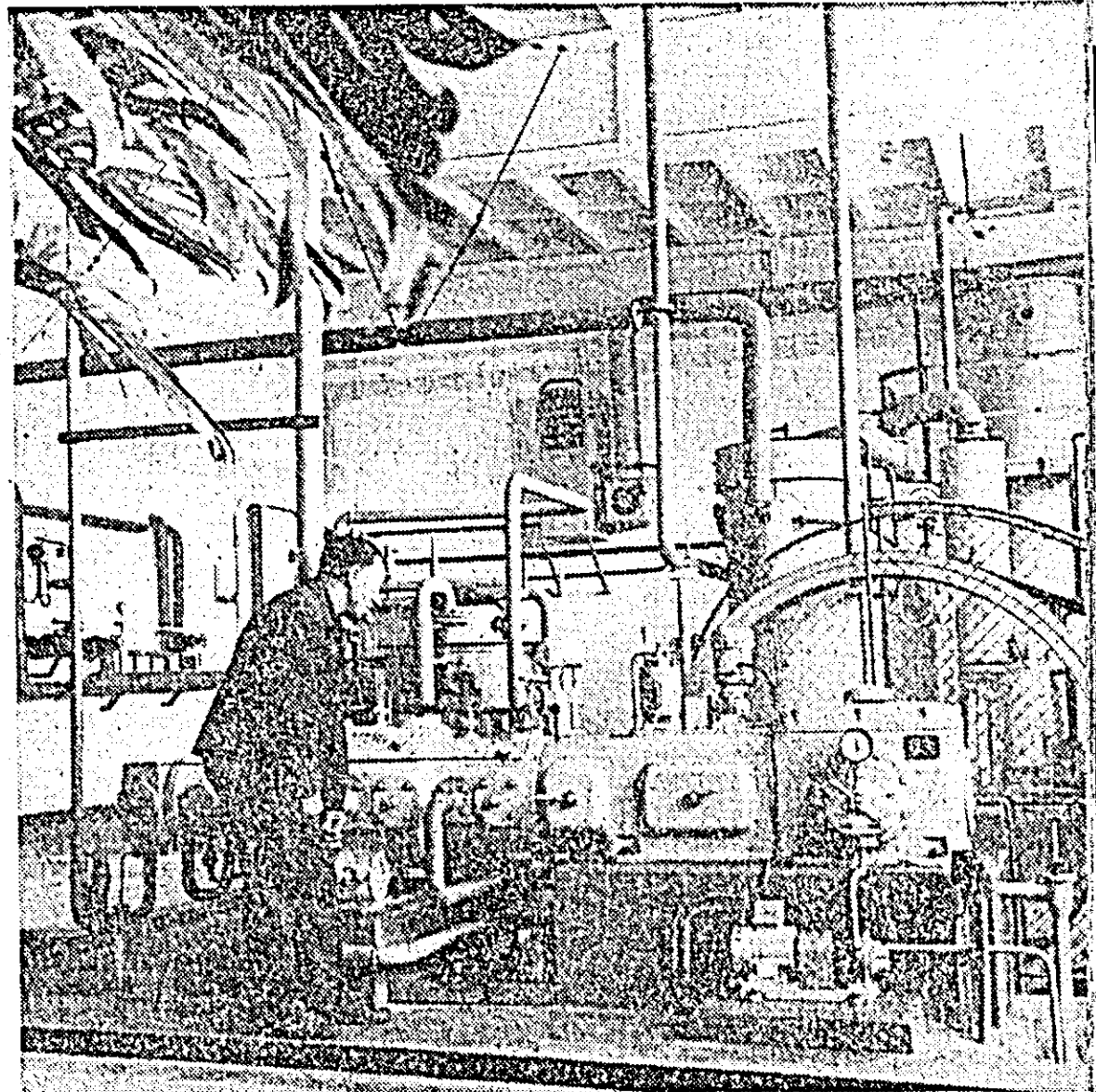
Aspect din interiorul fabricii de bloxid de carbon de la întreprinderea „7 Noiembrie”
