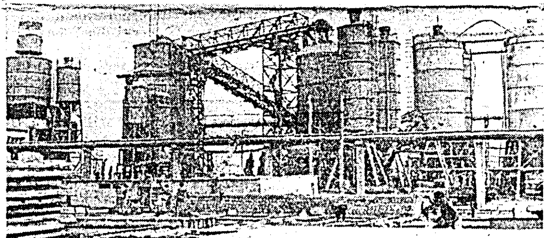
Aspect exterior al secției de prefabricate a I.C.M.J.
