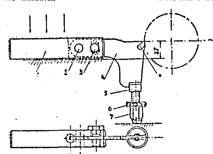
Cuțit de strînguns pentru strung, cu reazim
