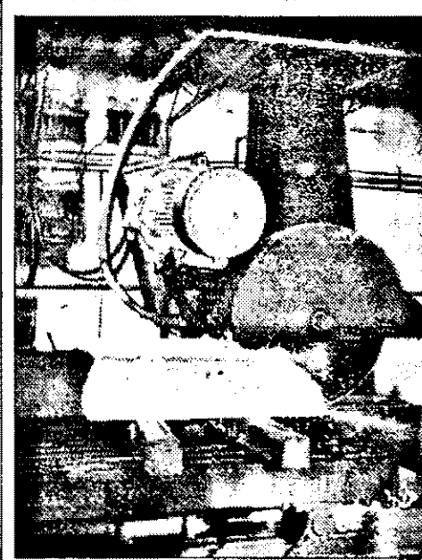
Debitarea unui bloc de marmură la circularul de 700 mm.
