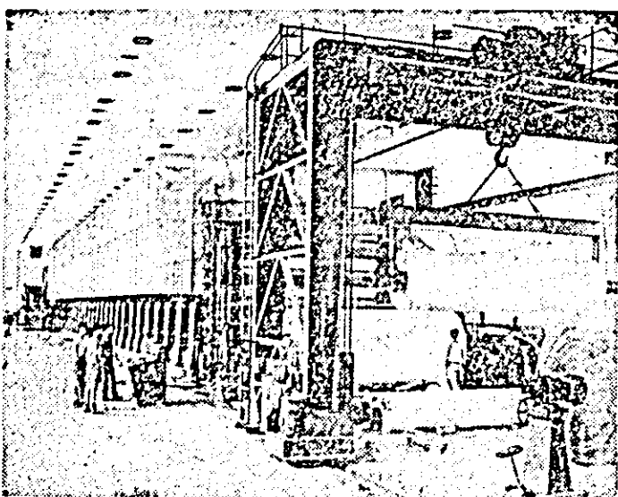
O secție a fabricii de hirtie din Guandun (Canton); în clădire: Mașina care produce 285 — 310 m hirtie de ziar pe minut în lățimea de 3,99 m.
