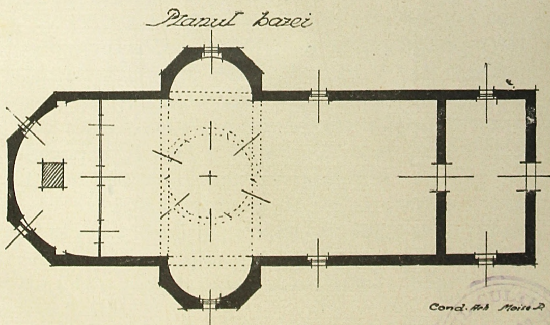
Biserica Mănăstirii Bodrog: secțiune și planul bazei
