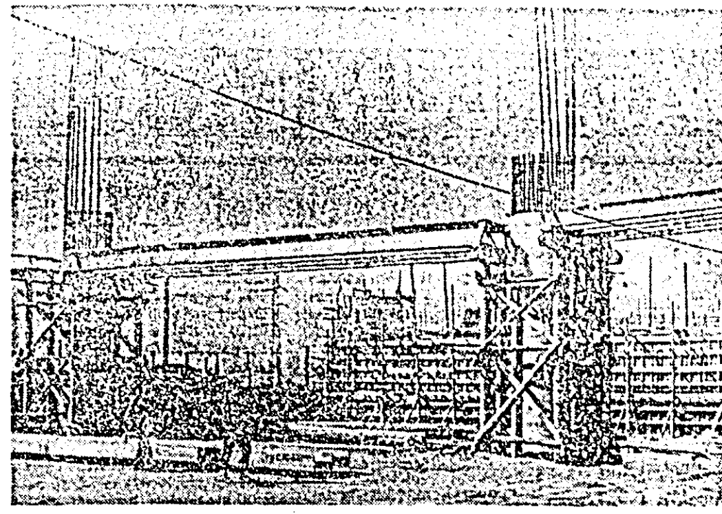
Se lucrează intens la pasarea de pe șoseaua Arad—București. Foto: A. POP
