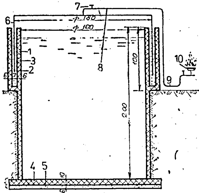
Schița instalației: 1. Cilindru interior (B 100); 2. — cilindru exterior (B 100); 3. Garnitură de apă; 4. Beton — B 100; 5. Balast; 6. Clopot din tablă; 7. Robinet; 8. Furtun din cauciuc; 9. Jeavă neagră Ø3,4 (oli); 10. Arzător (Dimensiunile sînt date în cm).
