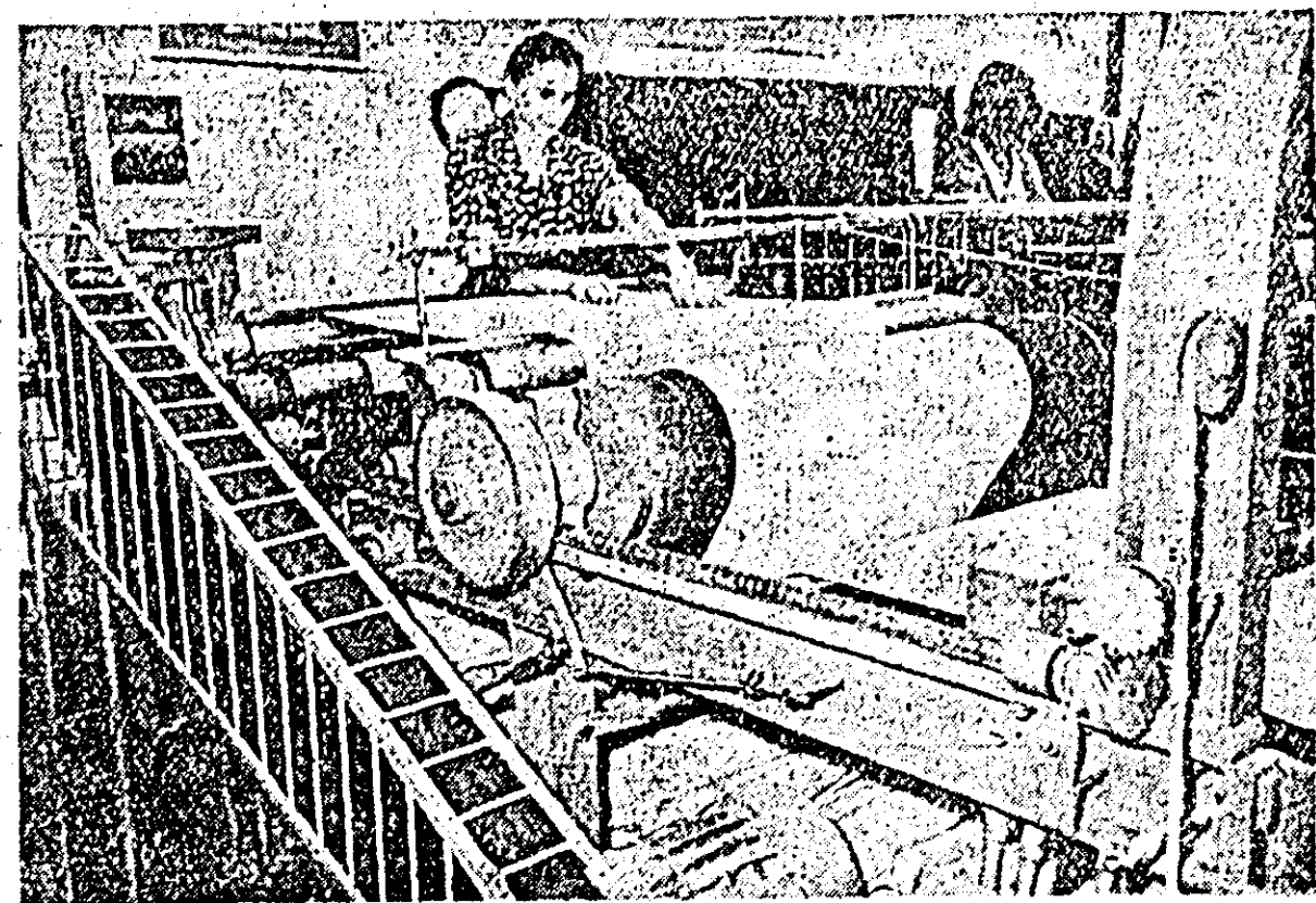
Secția catifea a uzinelor textile „30 Decembrie” s-a îmbogățit cu o nouă mașină de tăiat catifea. Aceasta a fost confecționată în întreprindere din resurse interne, după modelul celor existente în uzină. În clipă: noua mașină de tăiat catifea.
